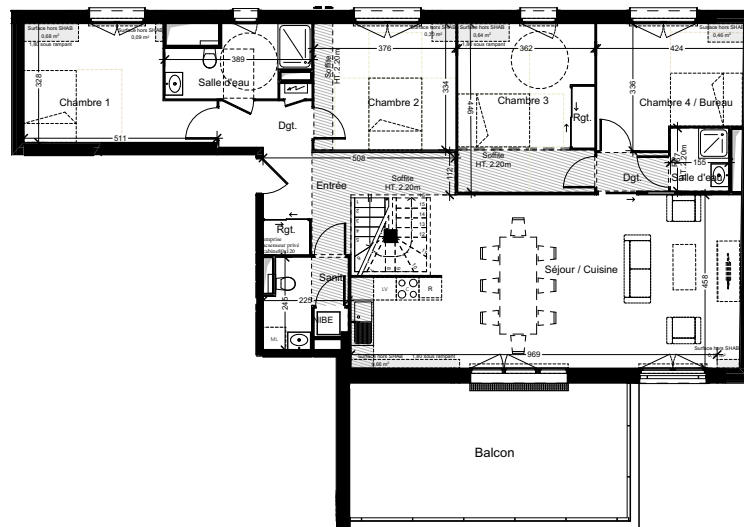
Comble niv 2
